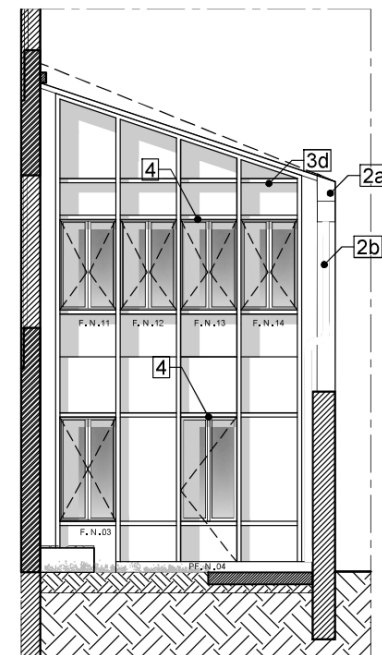
FAÇADE NORD
