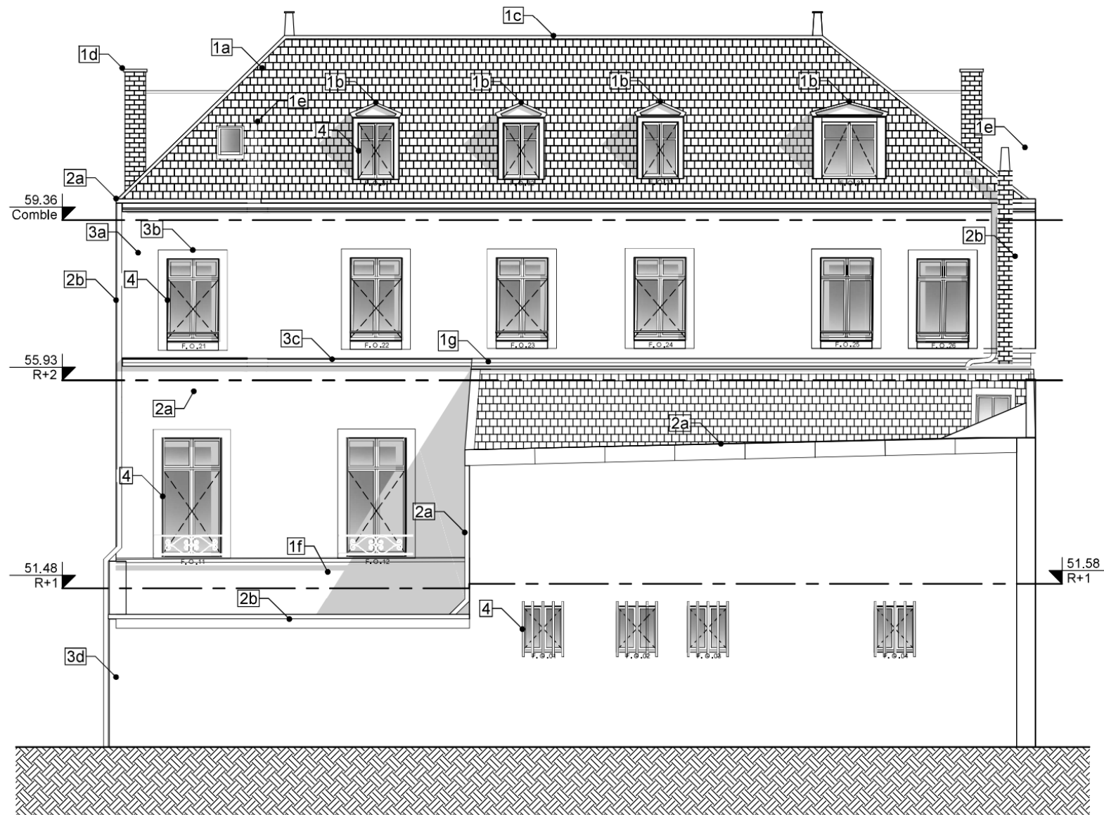
FAÇADE OUEST
